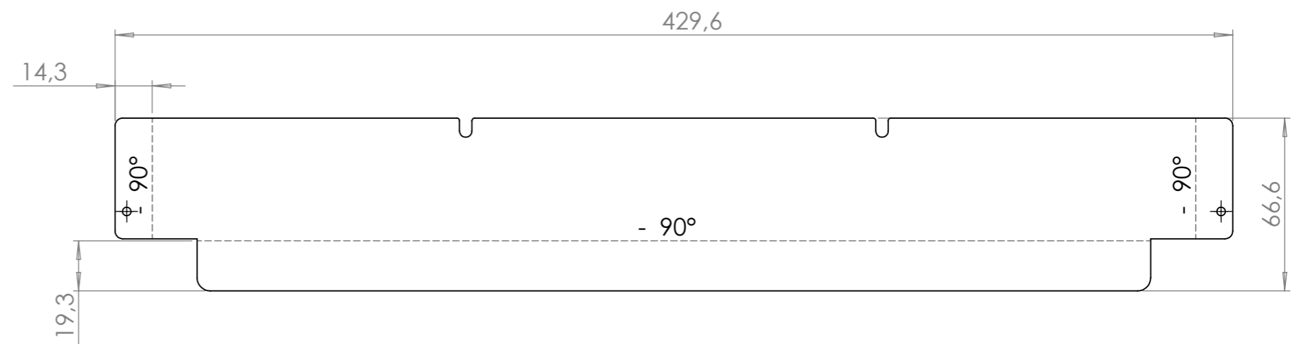
DETAIL B MAßSTAB 1 : 1
