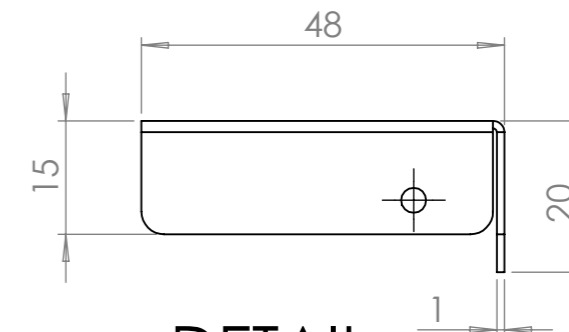
DETAIL B MAßSTAB 1 : 1
