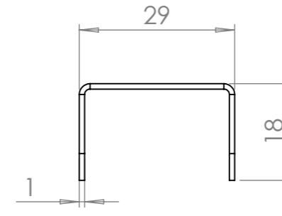
DETAIL A MAßSTAB 1 : 1
