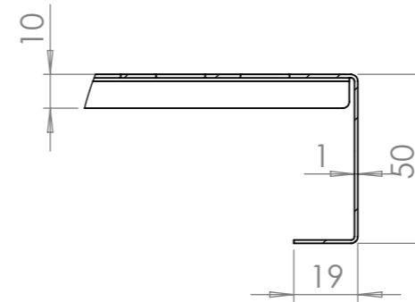
DETAIL E MABSTAB 1:2
